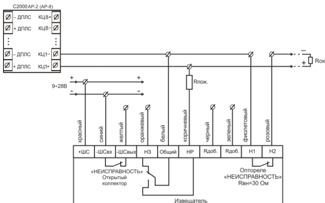
Рисунок 11 – 4-х проводная схема подключения Спектрон-204, -205 к C2000-AP2 (AP-8) с использованием режима «НЕИСПРАВНОСТЬ»
