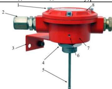
Рисунок 1. Внешний вид извещателя 1-винт М6 с шайбой; 2-кабельный ввод; 3-кронштейн; 4-гайка М30х1,5; 5-чувствительный элемент; 6-светодиодный индикатор; 7- корпус извещателя; 8- крышка извещателя.
