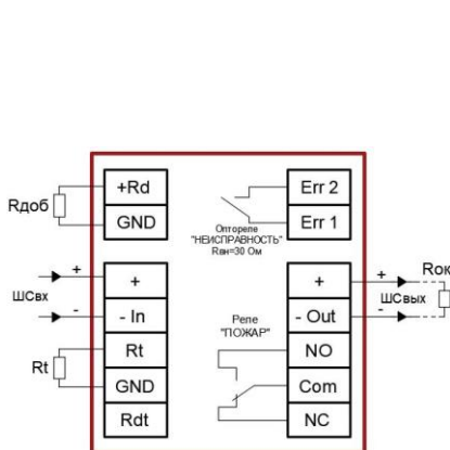
Рис.3 – Схема 2-х проводного подключения
