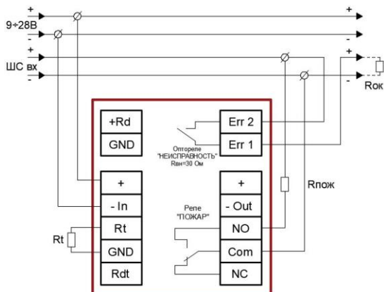
Рис.4 – Схема 4-х проводного подключения
