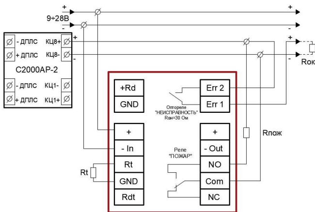
Рис. 5 – Схема подключения к адресному расширителю С2000-АР2 (АР8)
