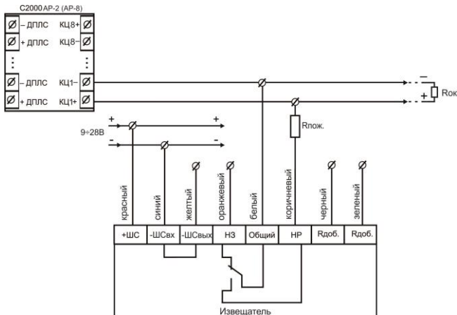
Рисунок 6 – 4-х проводная схема подключения к C2000-AP2 (AP-8) Спектрон-201P
