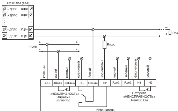
Рисунок 9 – 4-х проводная схема подключения к C2000-AP2 (AP-8) без использования режима «НЕИСПРАВНОСТЬ»
