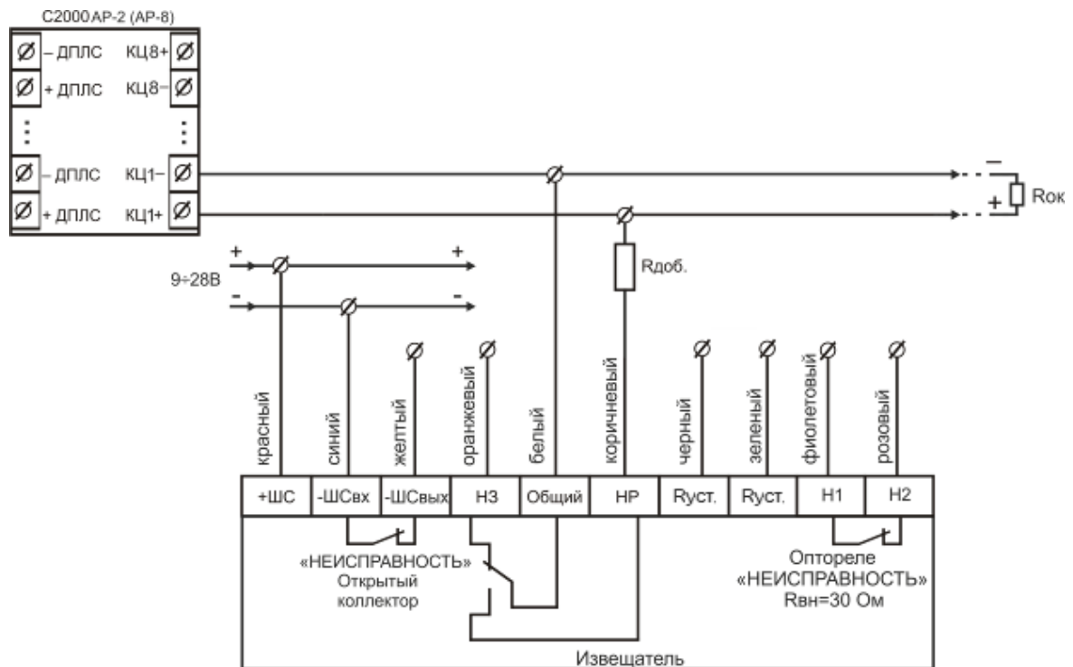
Рисунок 9 – 4-х проводная схема подключения к С2000-AP2 (AP-8) без использования режима «НЕИСПРАВНОСТЬ»
