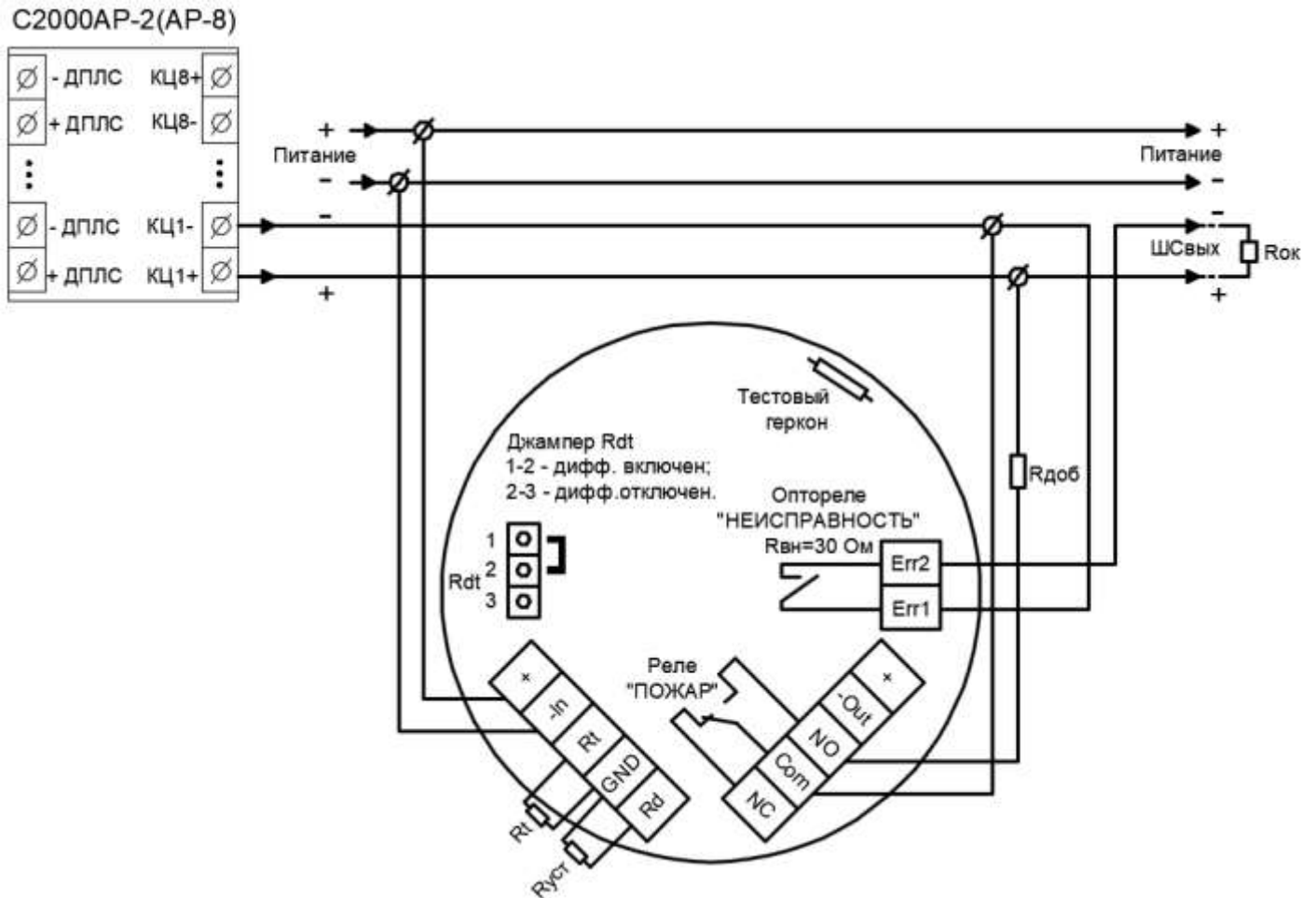
Рисунок 7 – 4-х проводная схема подключения к С2000-АР2 (АР-8)
