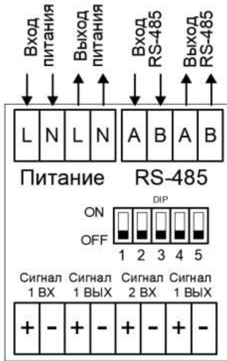
Рис. 5 Схема двухпроводного подключения оповещателя 220 В АС
