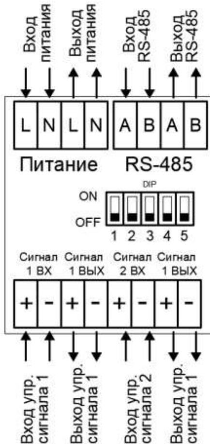
Рис. 6 Схема четырехпроводного подключения оповещателя 220 В АС
