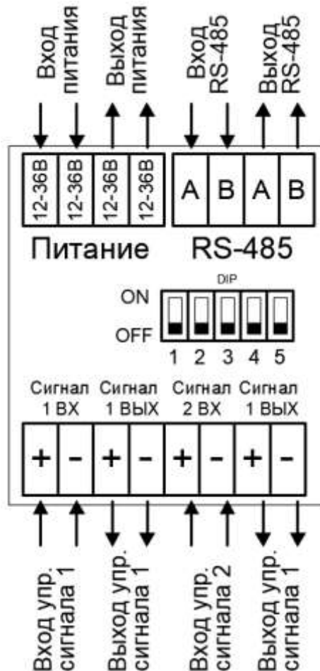
Рис. 4 Схема четырехпроводного подключения оповещателя 12-36 В DC
